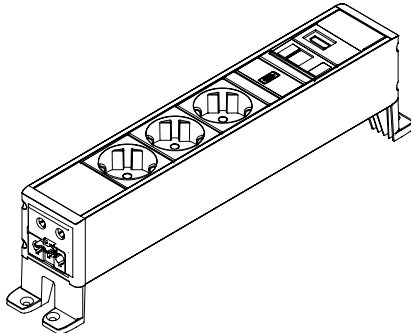
Electrificación Plus - carga rápida - para Top Access Doble (negro) Electrification Plus - fast charge - for Double top access (black) Electrification Plus pour Top-acces même finition que le plateau (noir) INCLUYE CONEXIÓN DE FUENTE DE ALIMENTACIÓN: INCLUDES POWER SUPPLY CONNECT: ALIMENTATION ÉLECTRIQUE INCORPORÉE: 3 SCHUKOS + USB CHARGE C INTELLIGENT CHARGE + RJ45 + 1 HDMI
