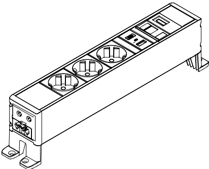
Electrificación Plus para Top Access Doble (negro) Electrification Plus for Double Top Access (black) Electrification Plus pour Top-acces même finition que le plateau (noir) INCLUYE CONEXIÓN DE FUENTE DE ALIMENTACIÓN: INCLUDES POWER SUPPLY CONNECT: ALIMENTATION ÉLECTRIQUE INCORPORÉE: 3 SCHUKOS + USB CHARGE A + C + RJ45 + 1 HDMI
